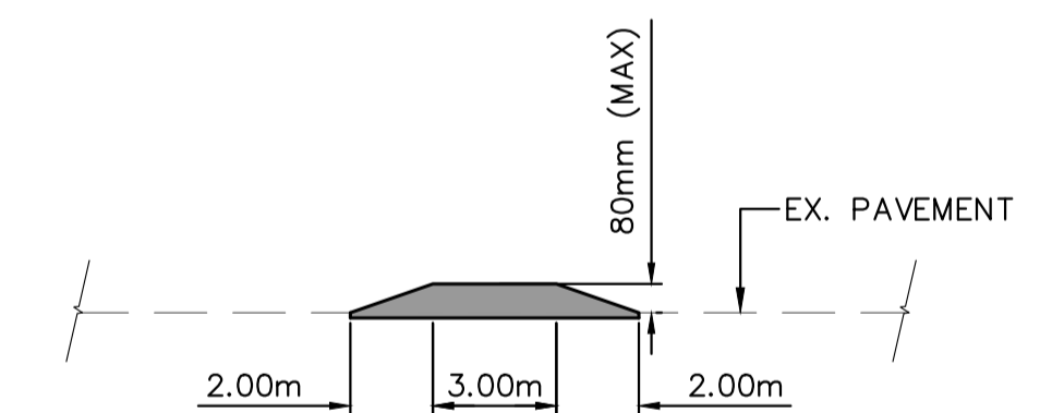
ROAD HUMP DETAIL 1:200 H N.T.S. V
